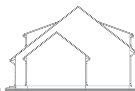
POHLED BOČNÍ PRAVÝ
