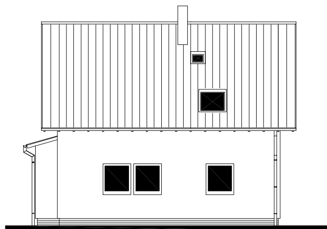
POHLED ZADNÍ
