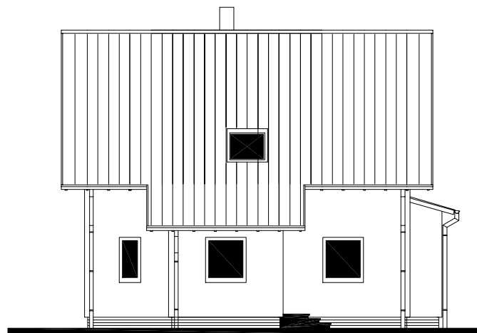
POHLED PŘEDNÍ
